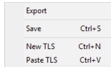
SSL menu
